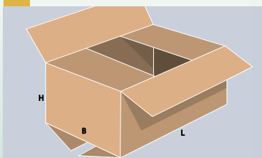
Faltkarton FEFCO 0201 mit zusammenstoßenden Boden-Deckel-Klappen
