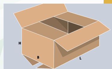
Faltkarton FEFCO 0201 mit zusammenstoßenden Boden-Deckel-Klappen
